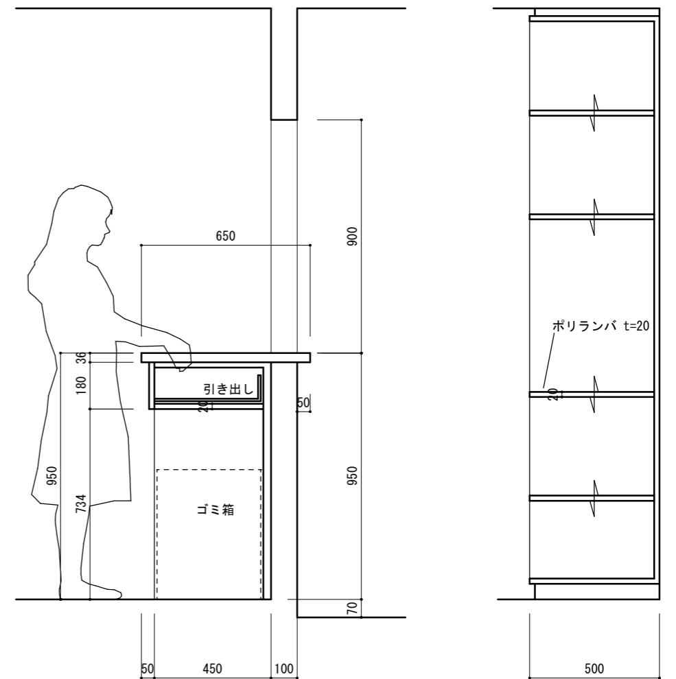
家具図C.D-2 1/20
