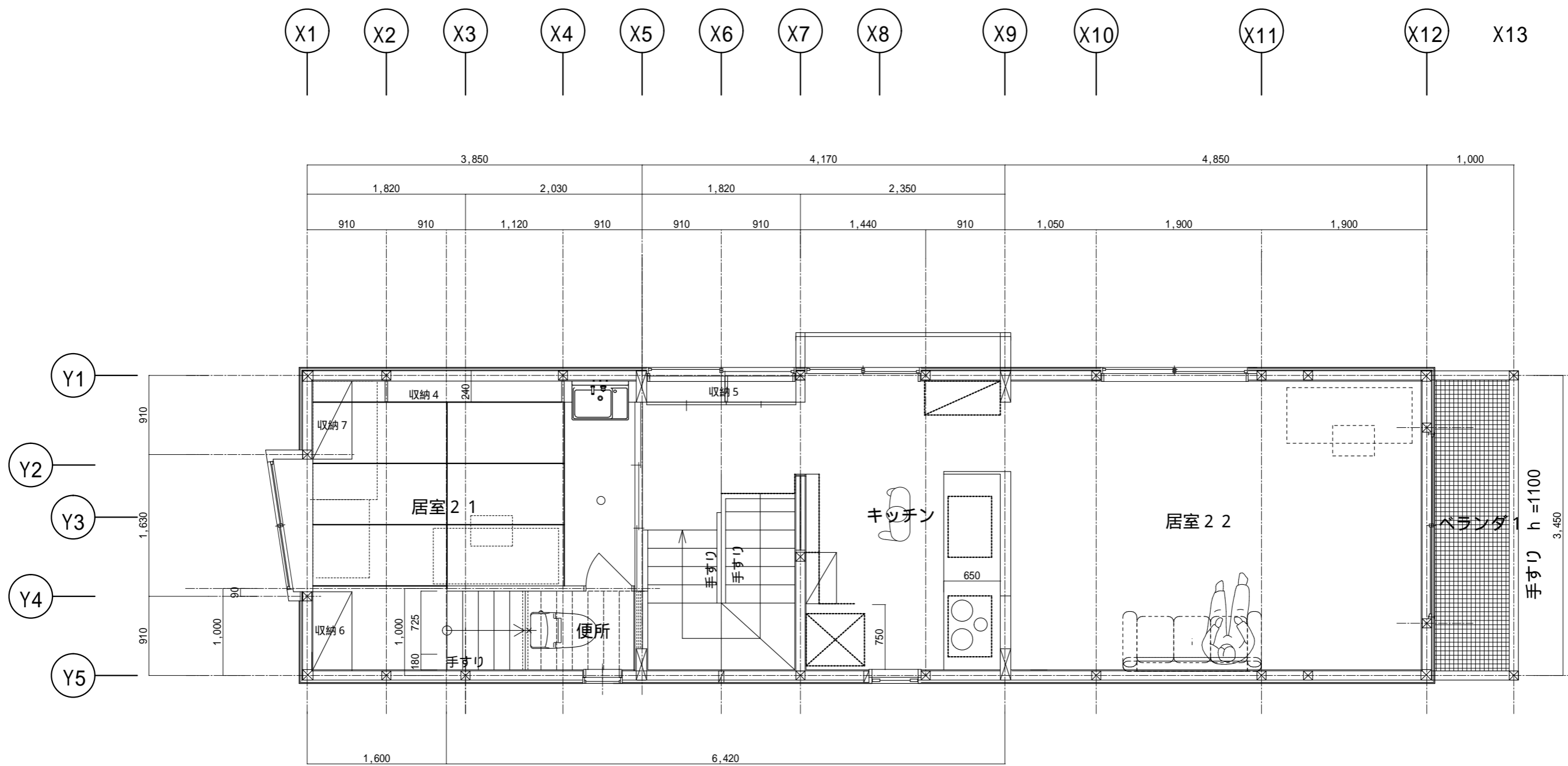
2階平面図 1 : 5 0
