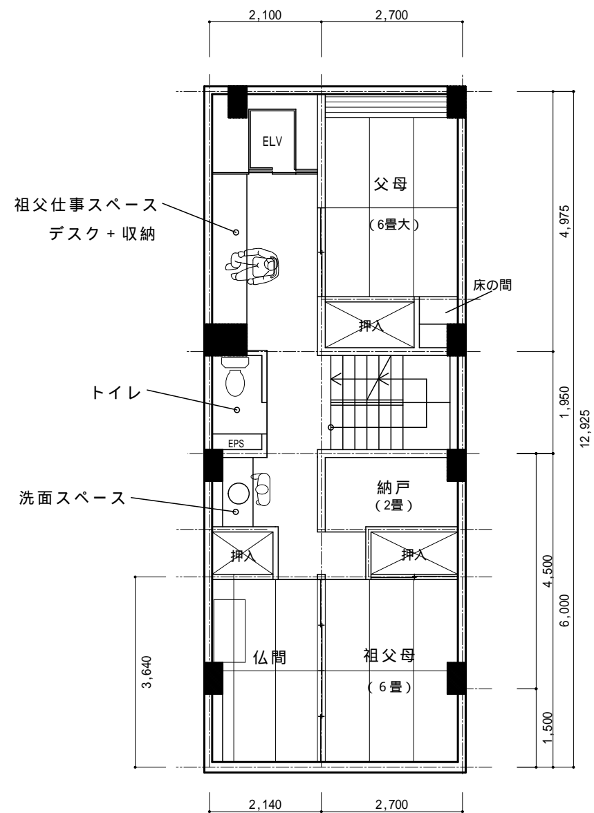
3階平面図
