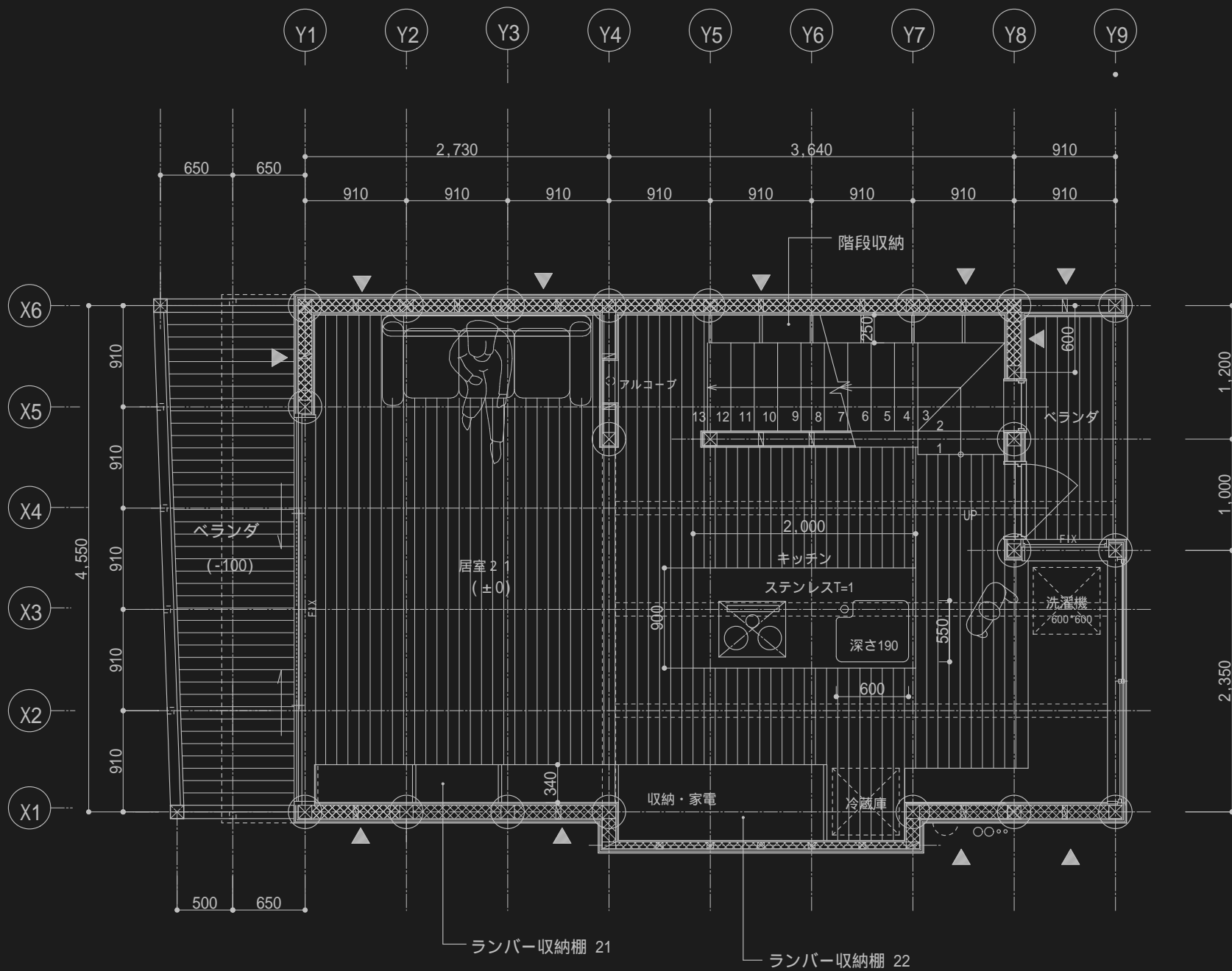
2F 平面図 1:50
