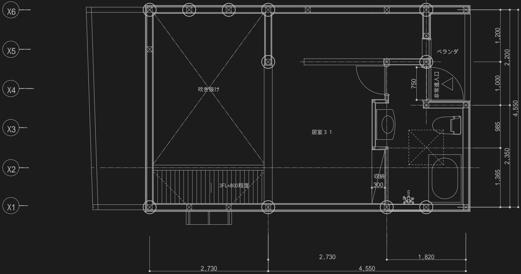
3F 平面図
