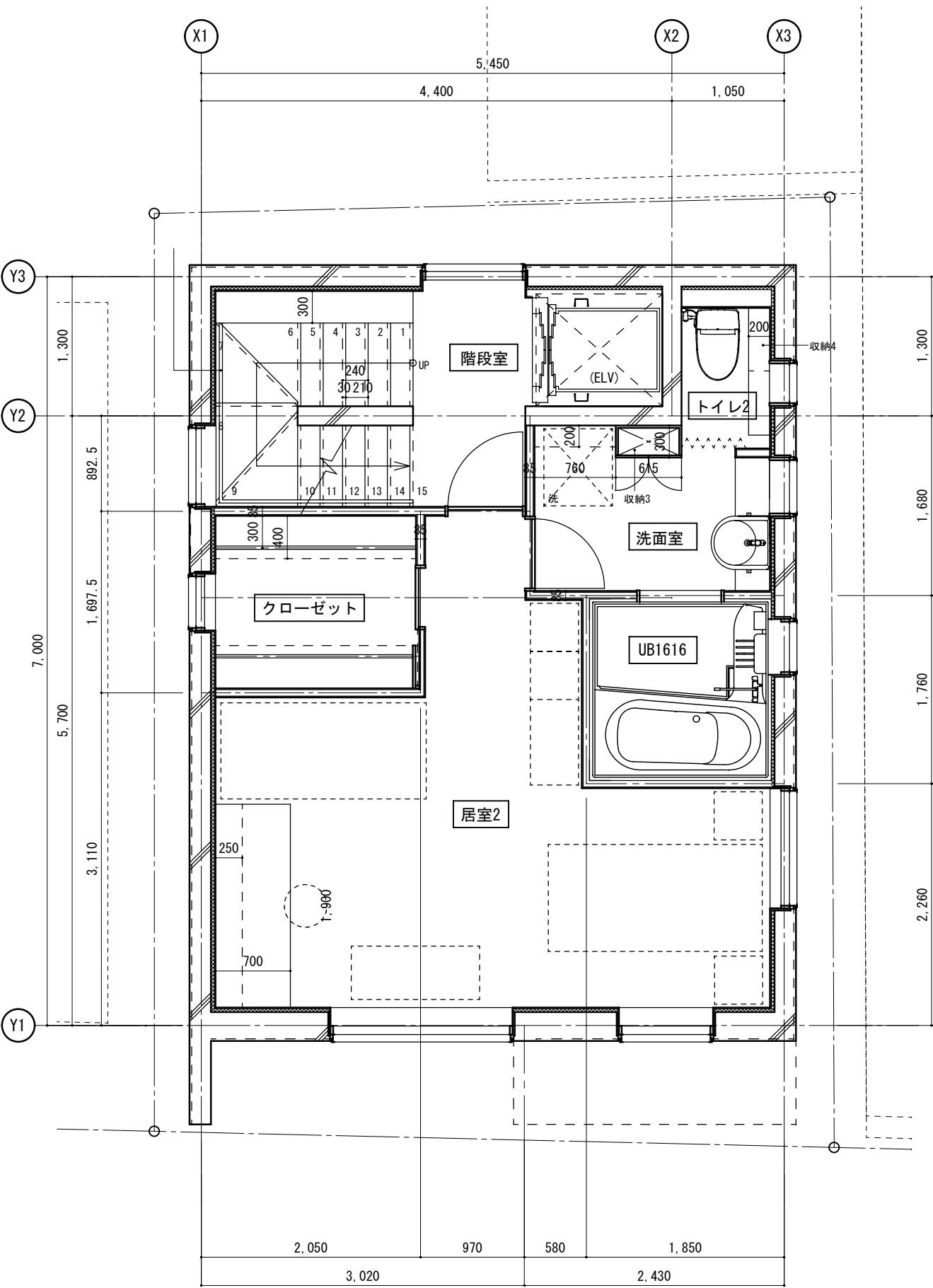
2階平面詳細図
