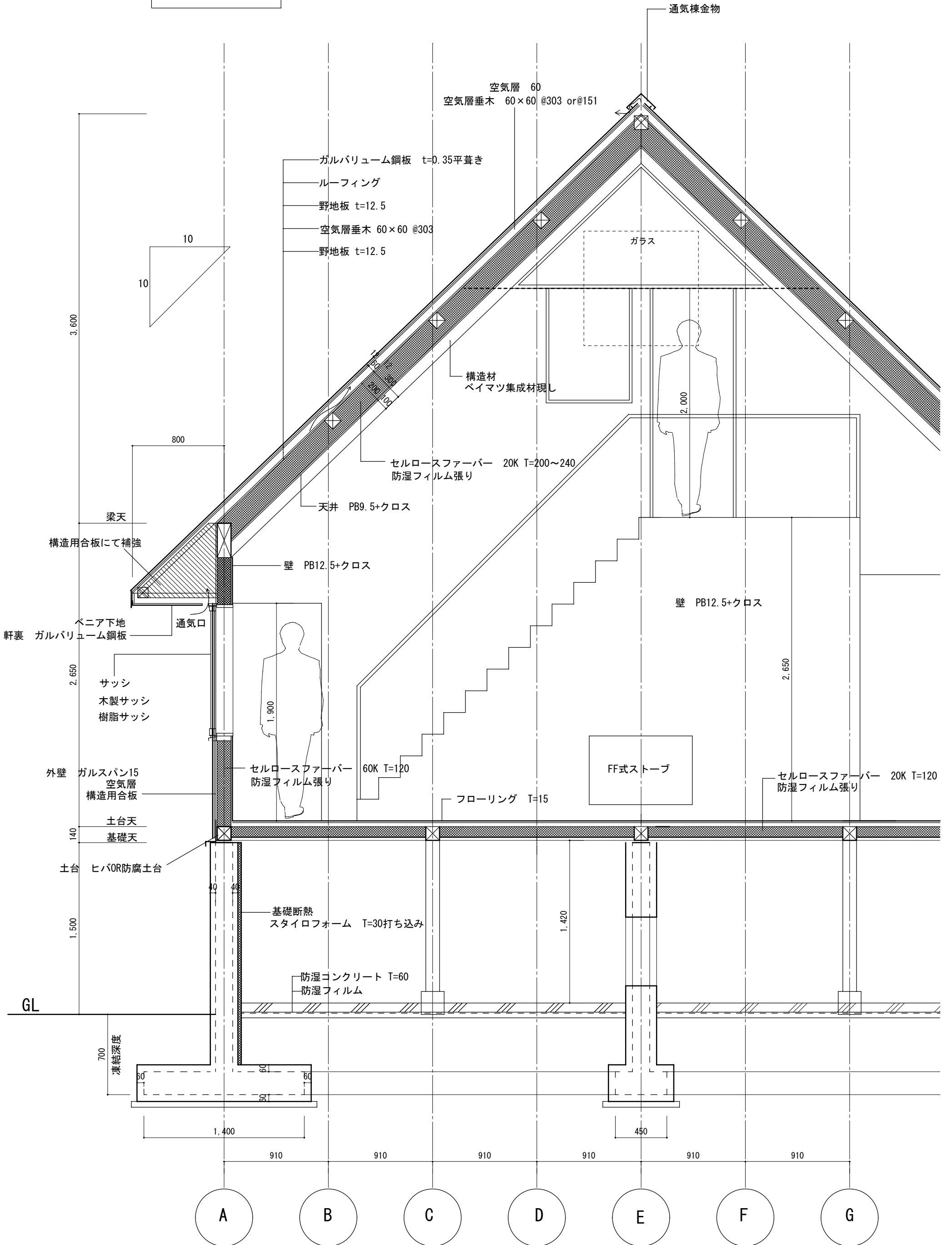
矩計図 1:30
