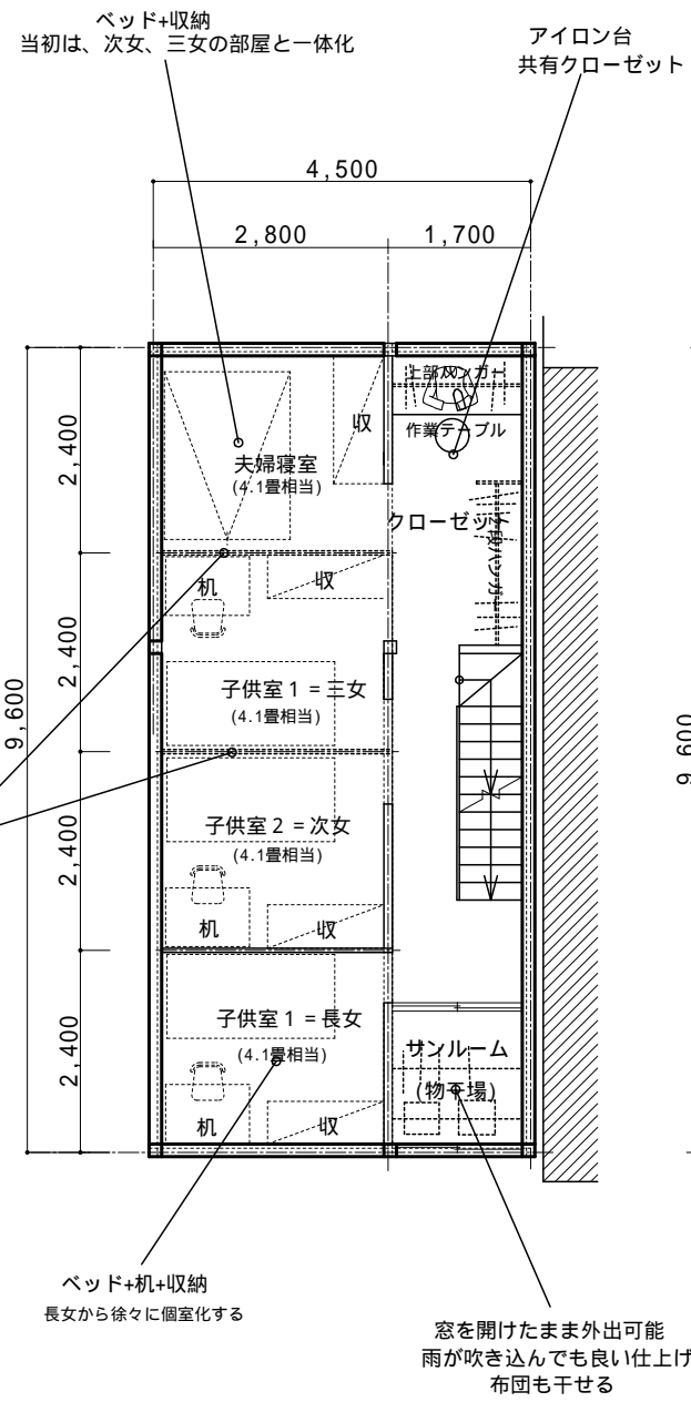
2階平面図
