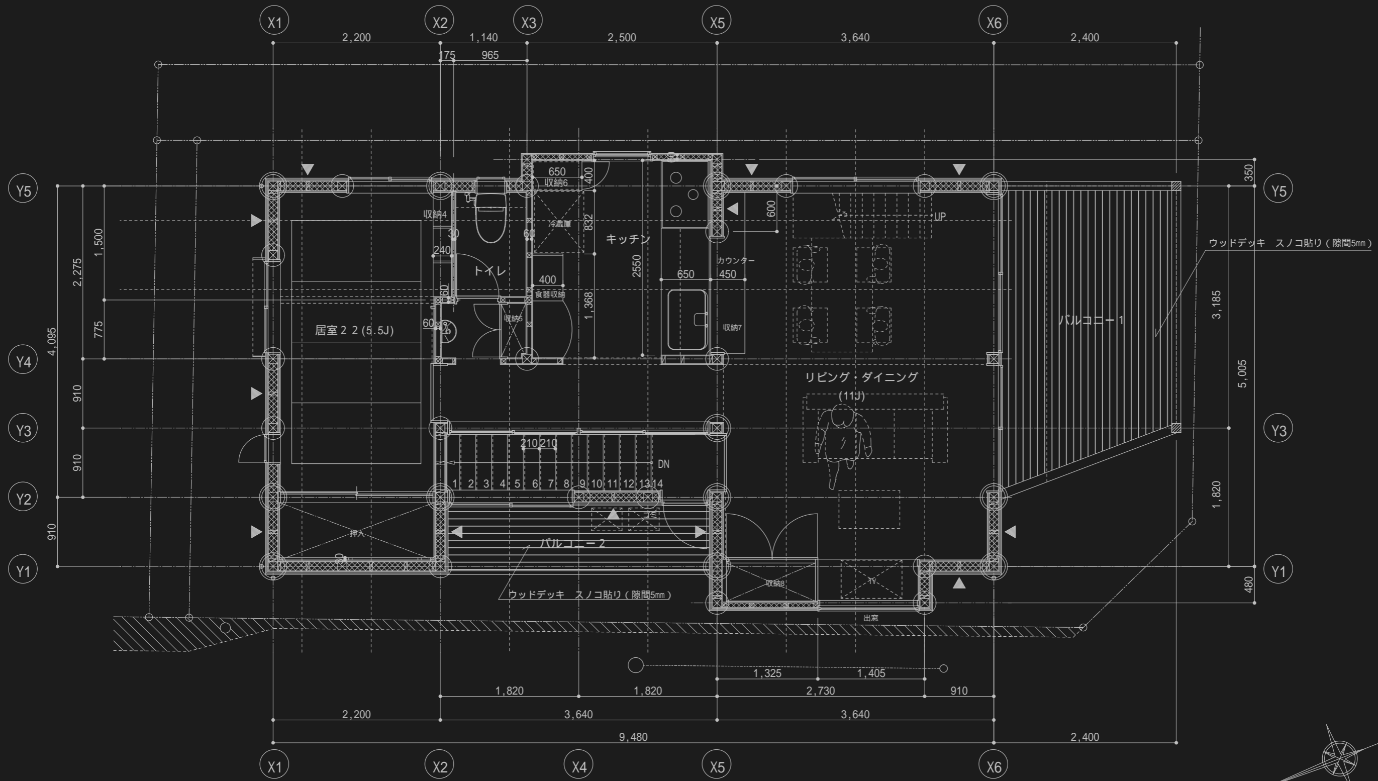
2階平面図
