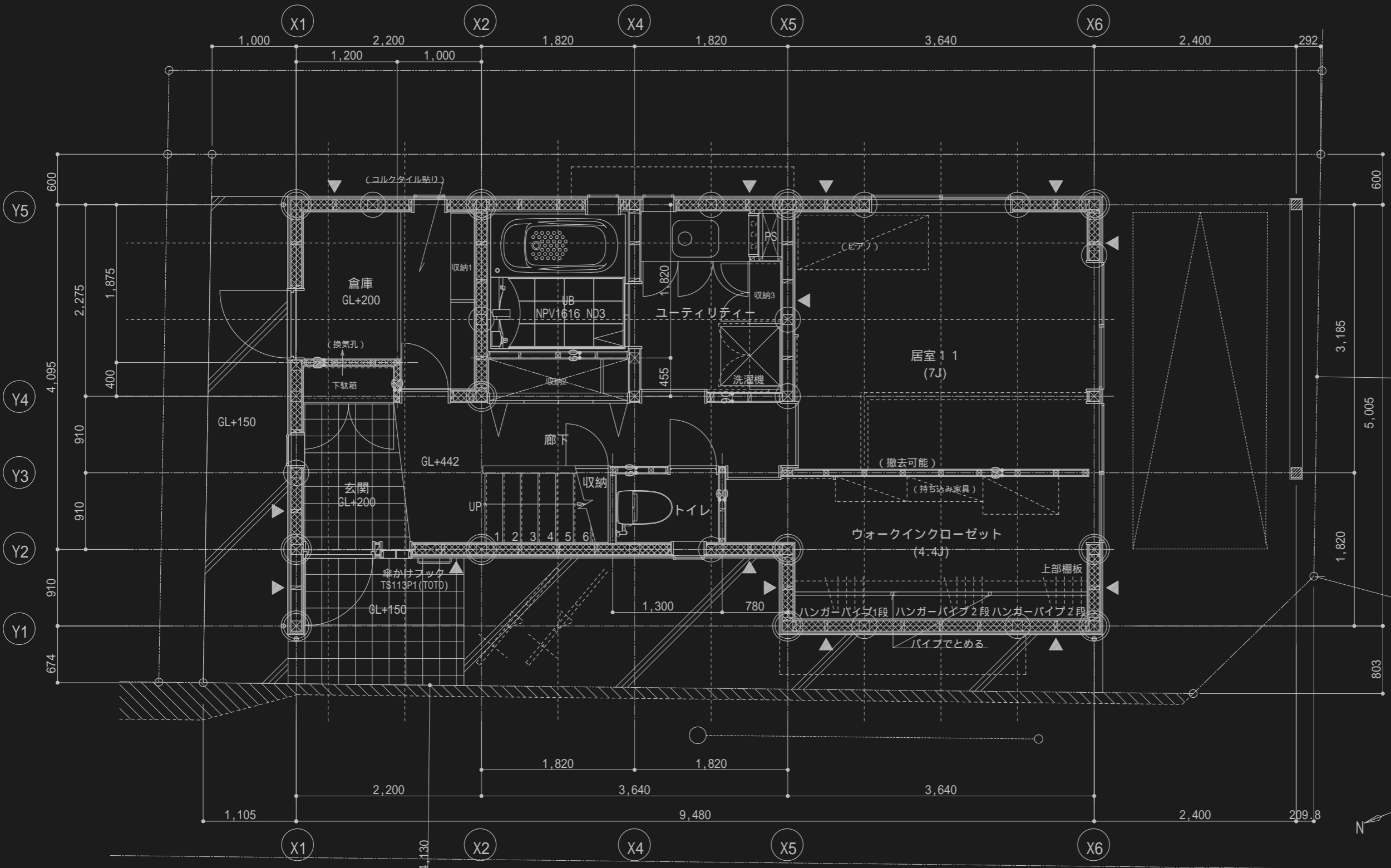
1階平面図
