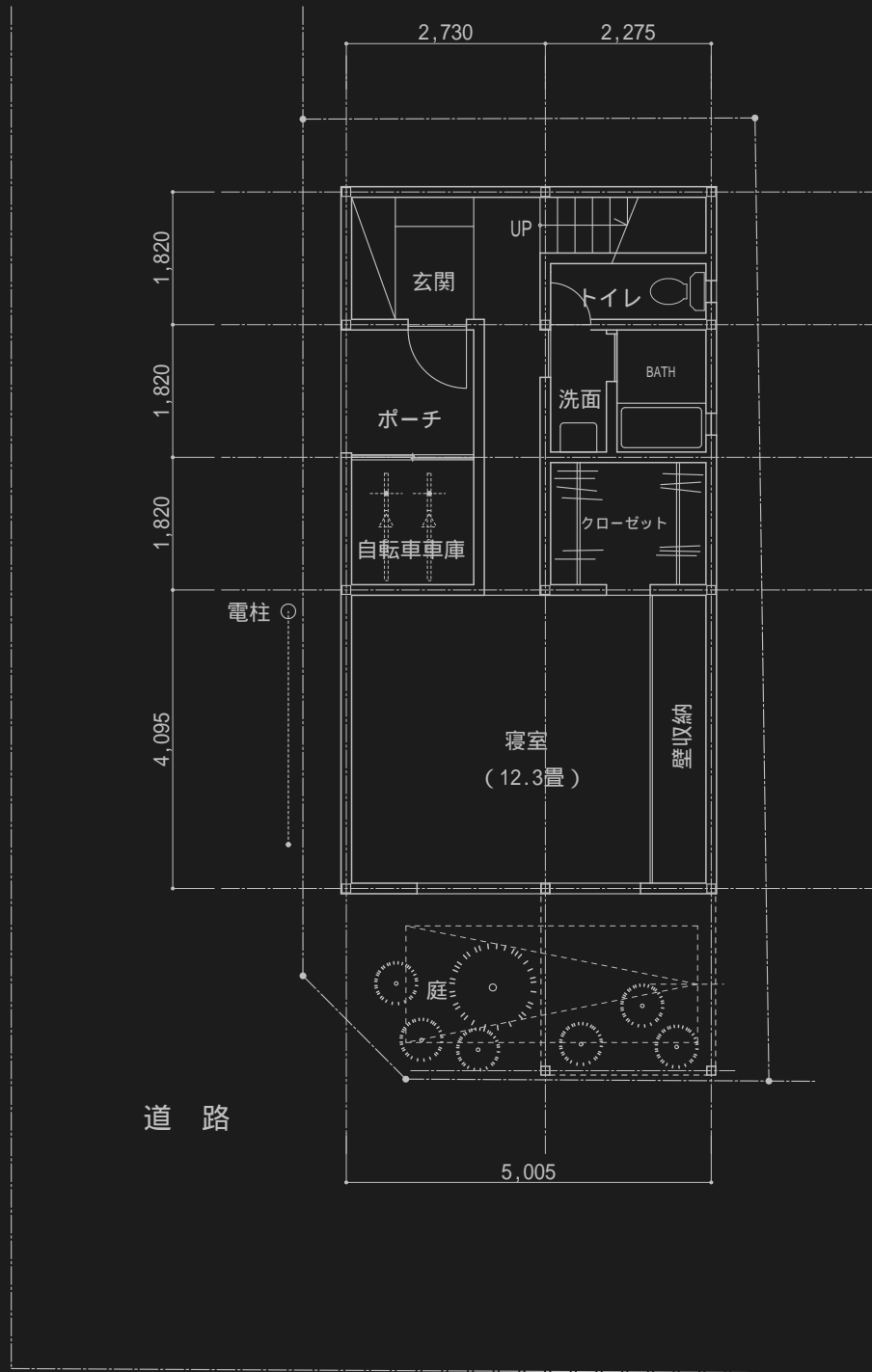
1F平面図 1/100
